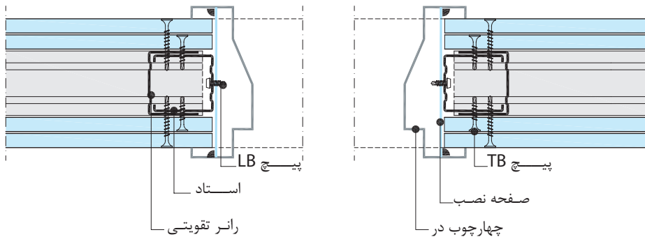
جزئیات نصب چهارچوب در (W112)
