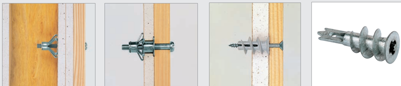
مهار جمع شونده فلزی (دیوار دو لایه)
